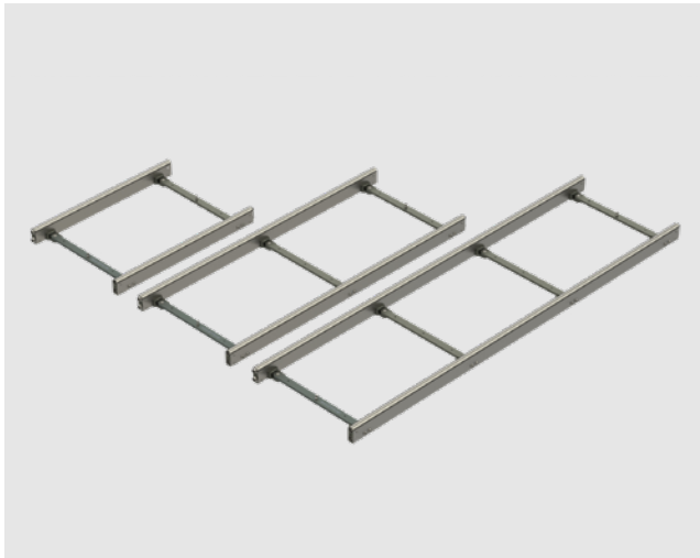
GF-Steel Track Spurweite 62/100 cm; Länge 90/160/230 cm
