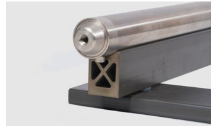
Verstärkter Unterzug als Kran Schiene
